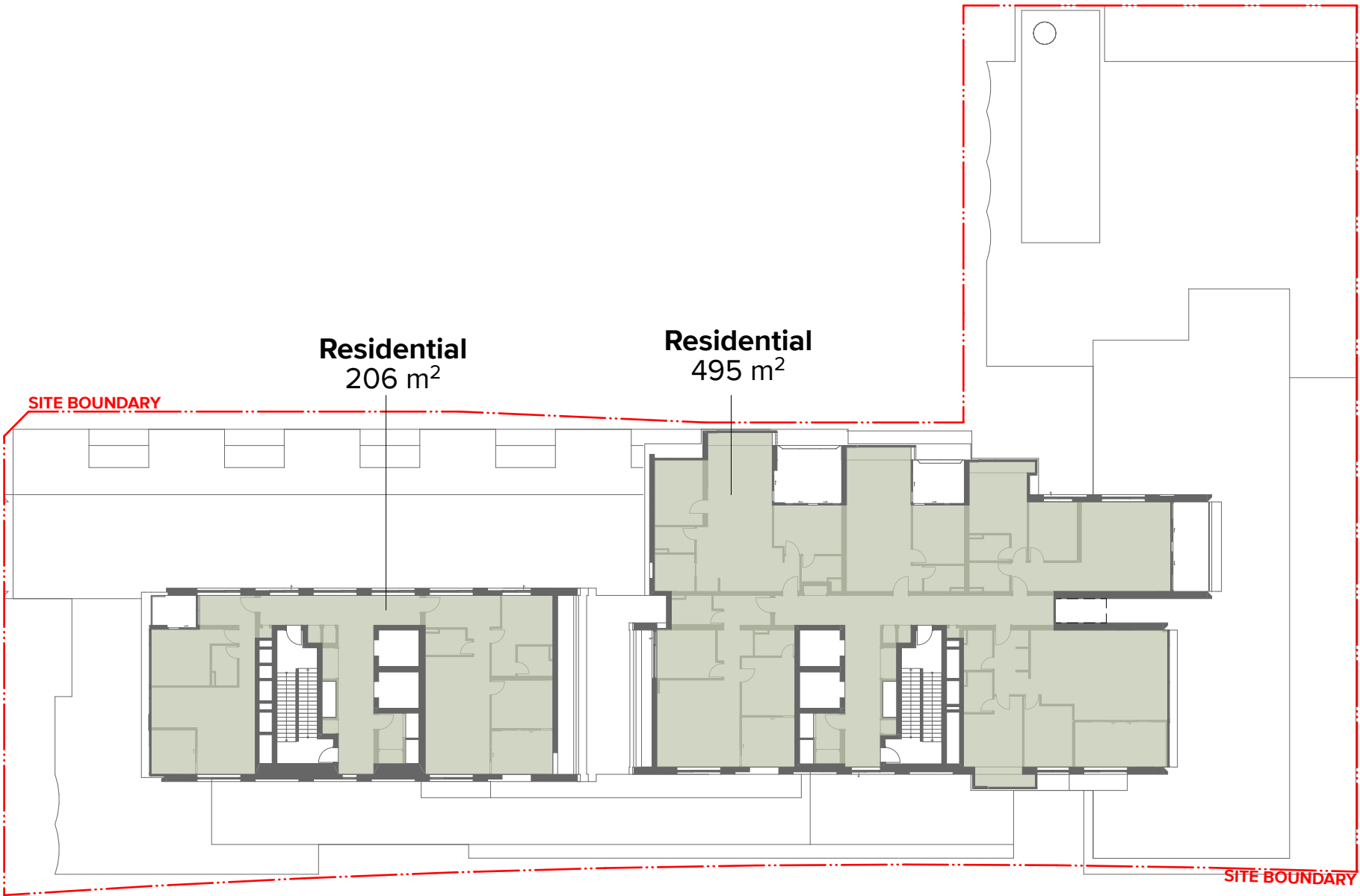
Level 11 GFA : 701m 2
