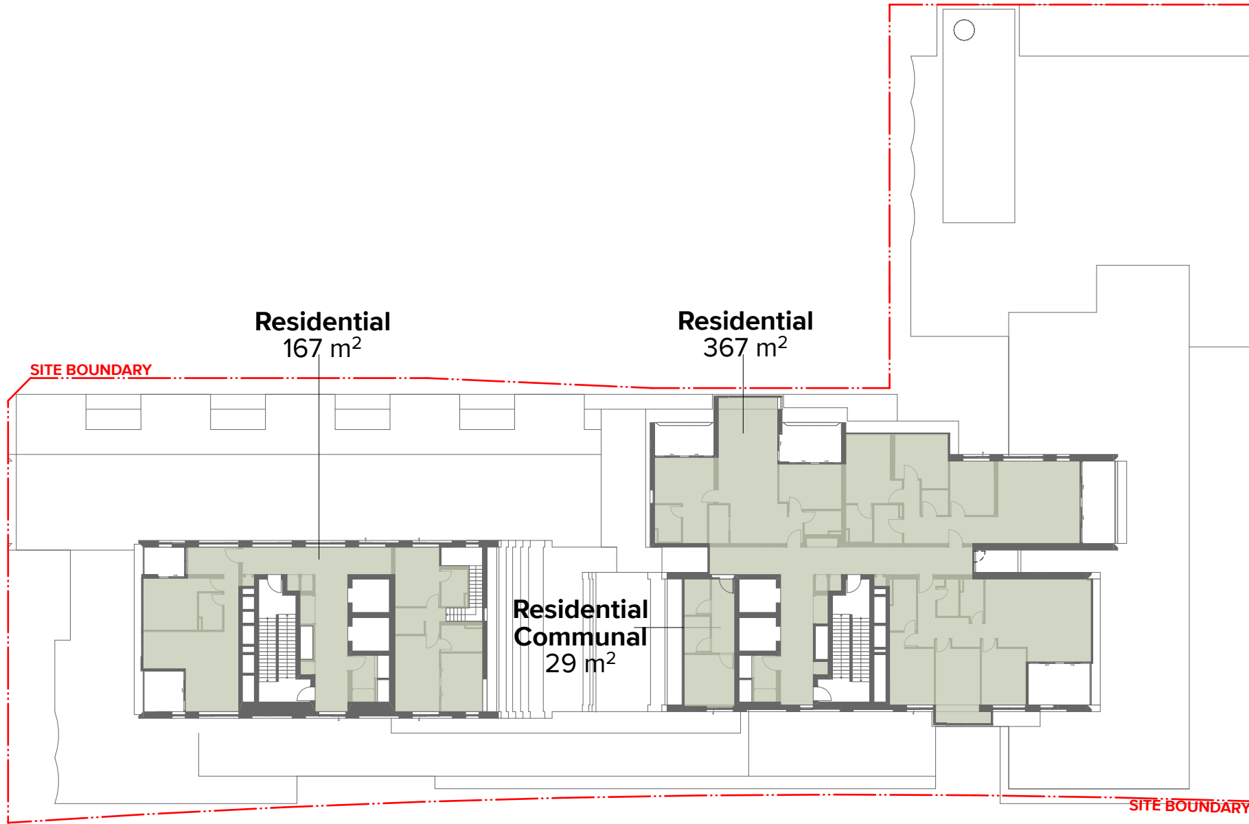
Level 16 GFA : 563m 2
